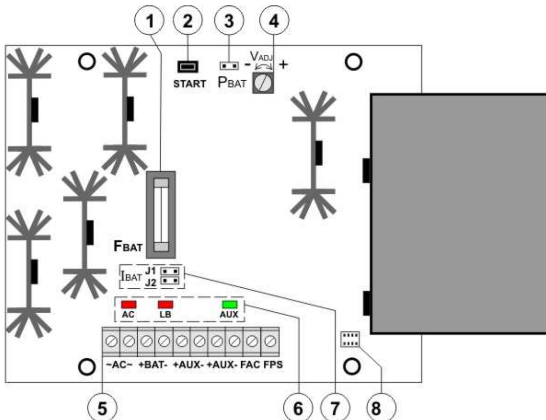
Rys. 2. Widok płyty pcb zasilacza.
