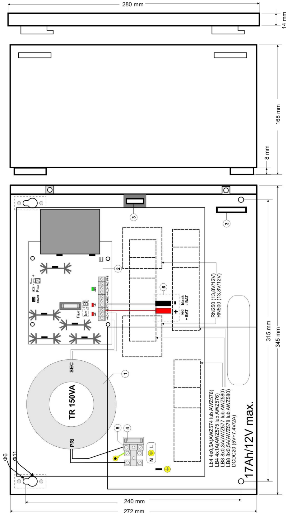
Rys.3. Widok zasilacza.
