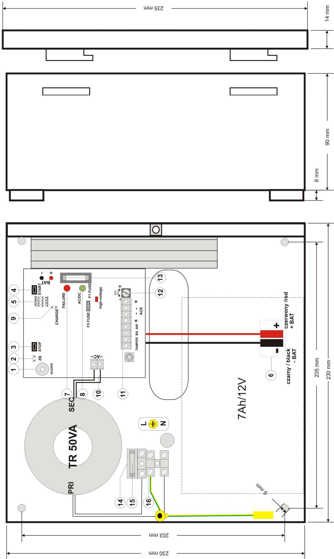
Rys.2. Widok zasilacza
