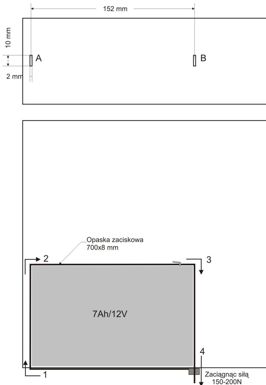
Rys.4. Procedura mocowania akumulatora.
