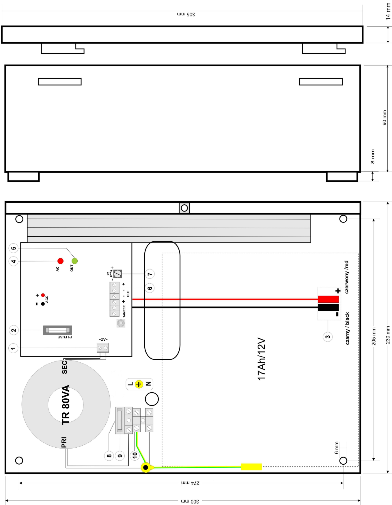
Rys. 3. Widok ogólny zasilacza.
