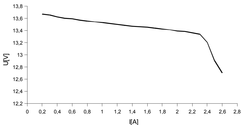
Rys. 2. Charakterystyka prądowo-napięciowa zasilacza.
