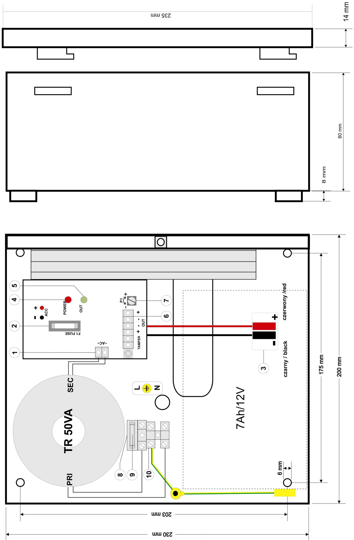
Rys. 3. Widok ogólny zasilacza.
